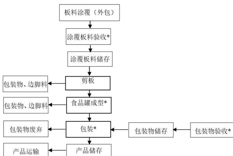
图 2.2 食品两片罐生产工艺流程图
